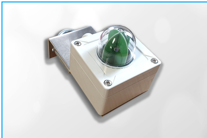
Abb. 1: Fotosensor FO-4 inkl. Montagewinkel
